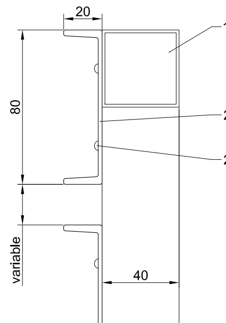
Detalle sección
